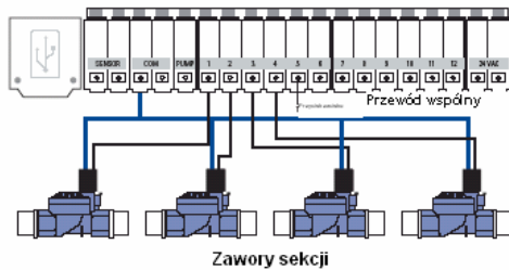
Rysunek 5: Podłączenie przewodu zraszacza
